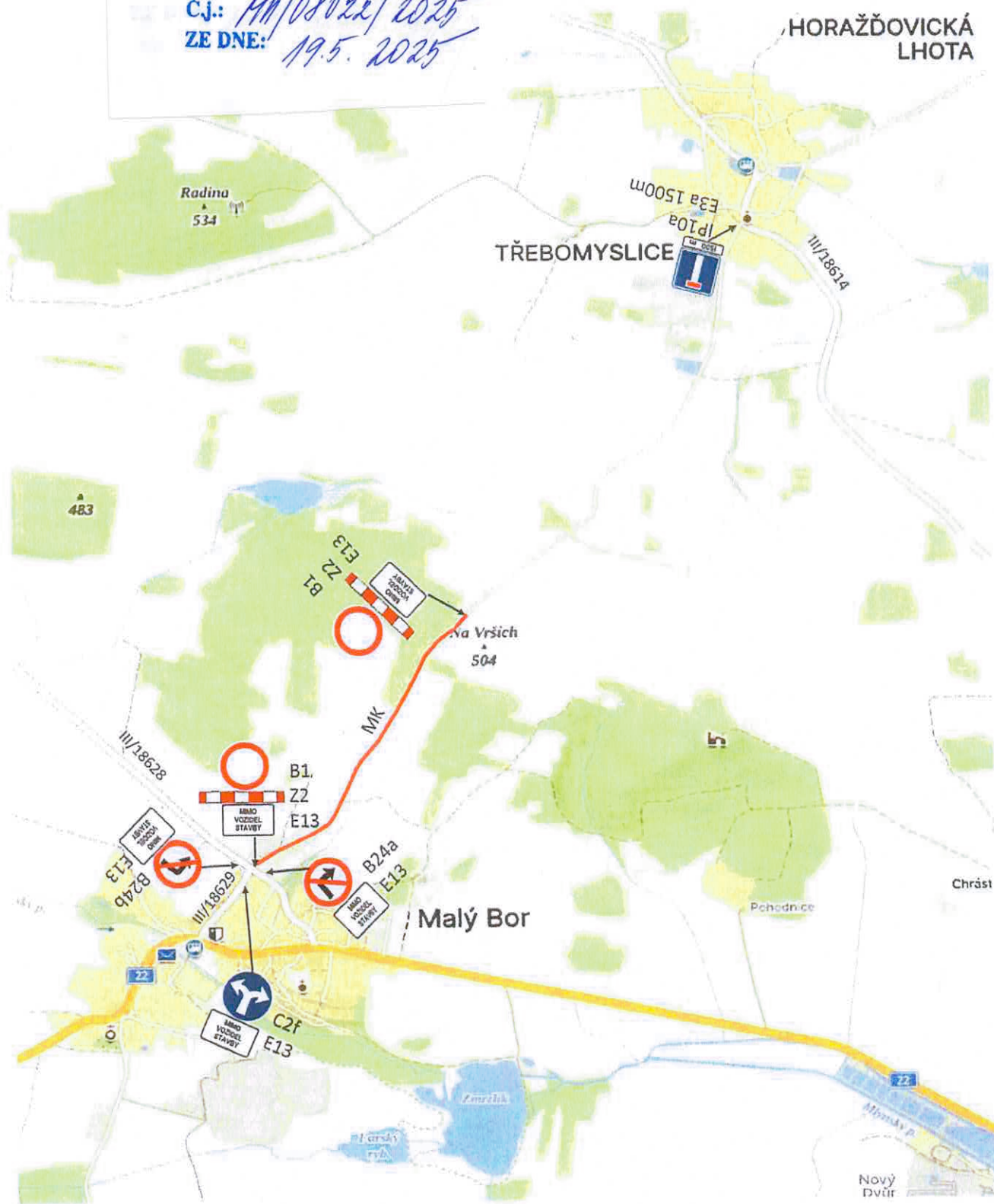
Oprava místní komunikace Malý Bor - Třebomyšlice - návrh přechodné úpravy provozu na PK
